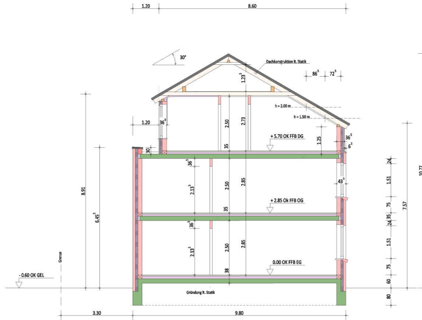
Querschnitt B - B
