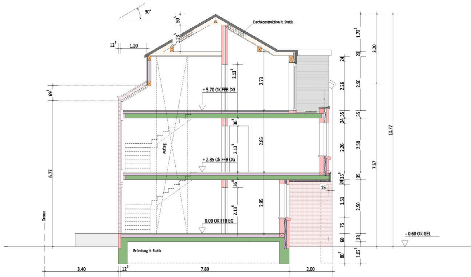
Querschnitt A - A
